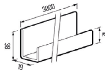
FS - 251 moldura universal
