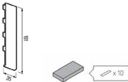
J - 201 tapa de junta para FS -201
