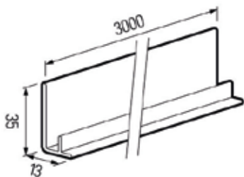
FS - 211 moldura de inicio
