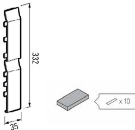
J - 202 tapa de junta para FS -202
