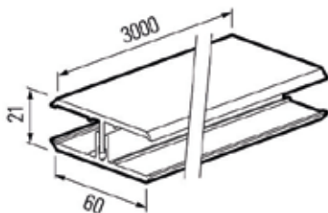
FS - 282 conector (2 piezas)
