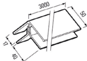
FS - 222 esquina universal (2 piezas)
