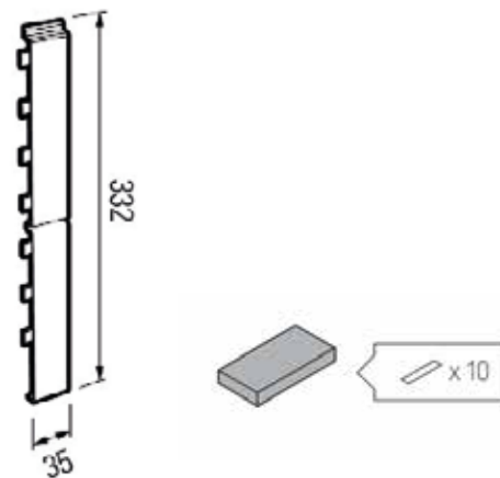
J - 302 tapa de junta para FS - 302
