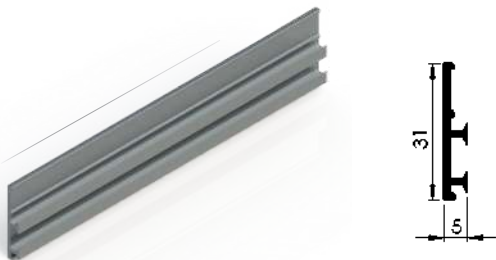
PERFIL CLIP FIJO PA CLIP PROFILE FIX PA SYSTEM
